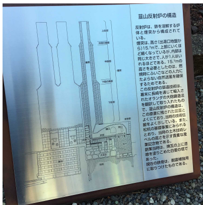
写真5 反射炉の図説 写真6 炉床と出湯口 写真7 作られた大砲 株式会社TOSEIの本社に向かい、変貌した会社の概要説明と新工場を見せてもらいました。
